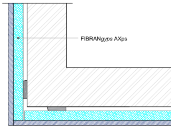
PART. 3 RACCORDO AD ANGOLO ESTERNO
