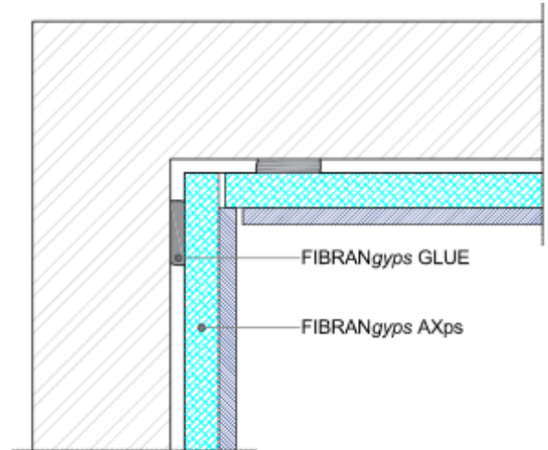
PART. 2 RACCORDO AD ANGOLO INTERNO
