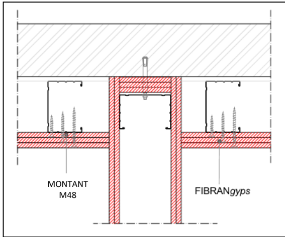
Part. 1 Intersection à cloison coupe-feu
