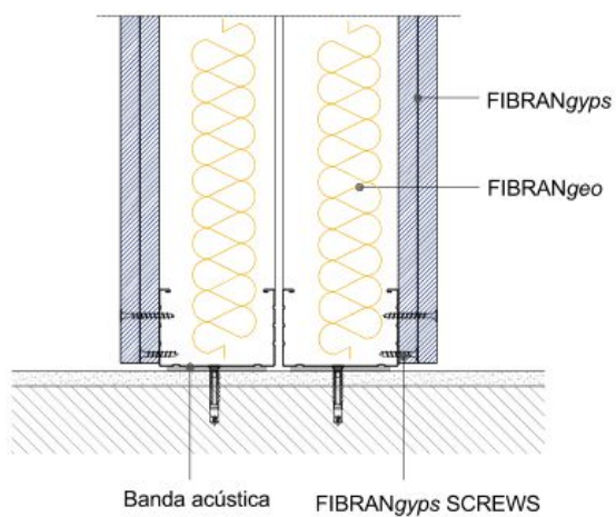
Det. 5 CORTE VERTICAL
