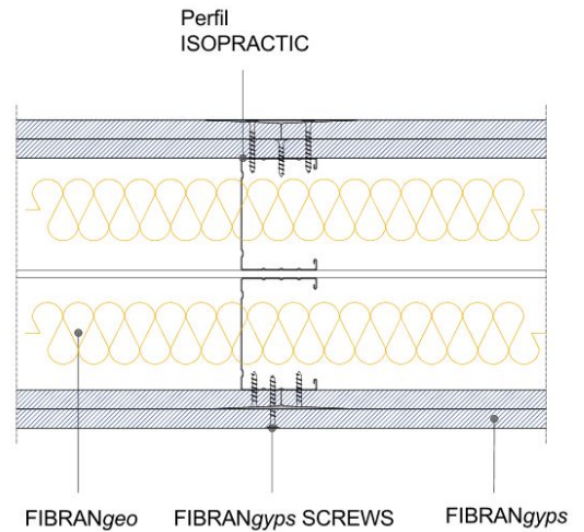
Det. 2 COLOCACIÓN DE LA DOBLA PLACA
