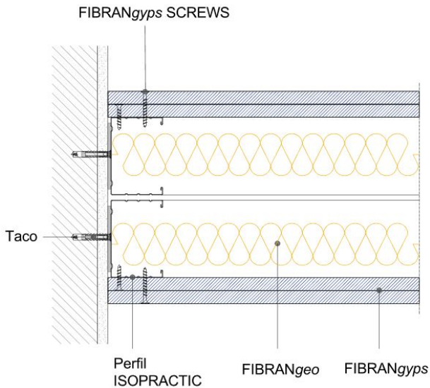
Det. 1 CONEXIÓN A LA PARED
