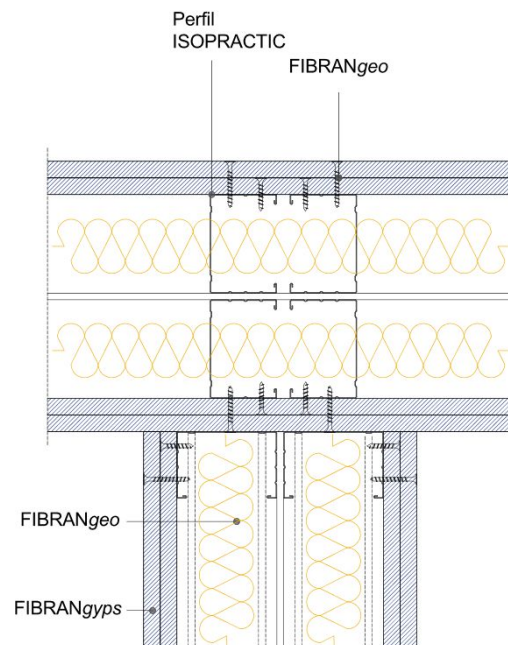
Det. 4 CONEXIÓN A "T"
