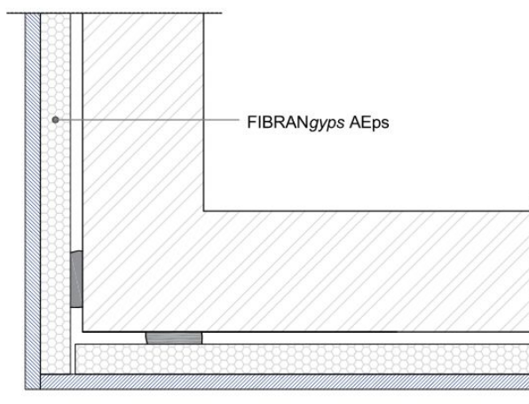
Det. 3 CONEXIÓN A "L" EXTERIOR
