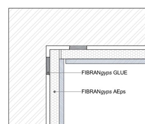
Det. 2 CONEXIÓN A "L" EN INTERIOR
